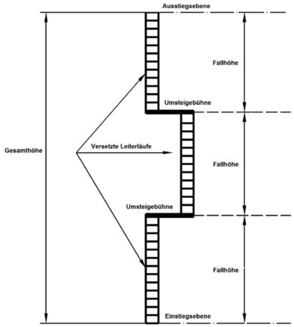
Abb. 5 Mehrzügige Steigleiter
