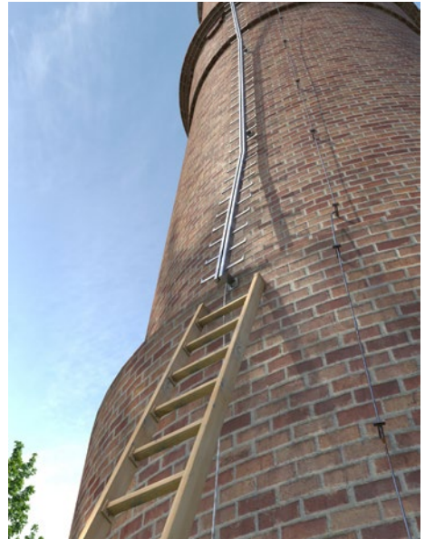
Abb. 13 Unsichere Zugangssituation bei Steigleitern an Schornsteinen
