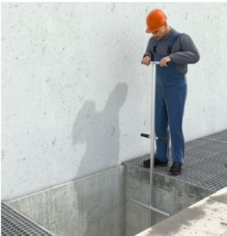
Abb. 17 Mobile Haltevorrichtung Quelle: Fa. Günzburger Steigtechnik
