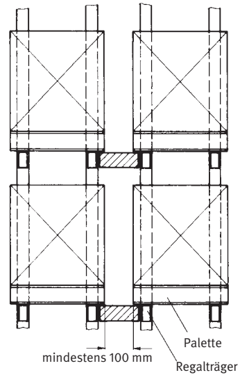
Abb. 8b: Sicherheitsabstand
