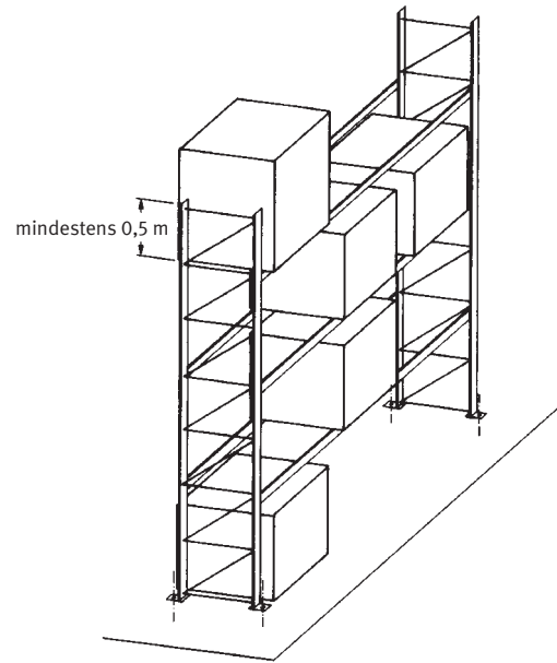
Abb. 7: Beispiel einer Sicherung gegen seitliches Herabfallen der Ladeeinheiten
