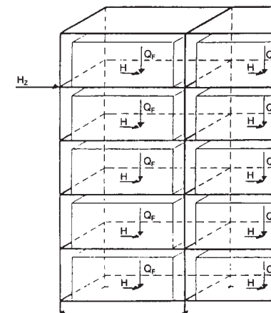
Abb. 1: Höchstzulässige Durchbiegung der tragenden Elemente von Lagereinrichtungen
